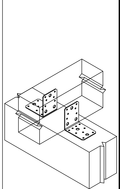
Instalação para 2 esquadros
