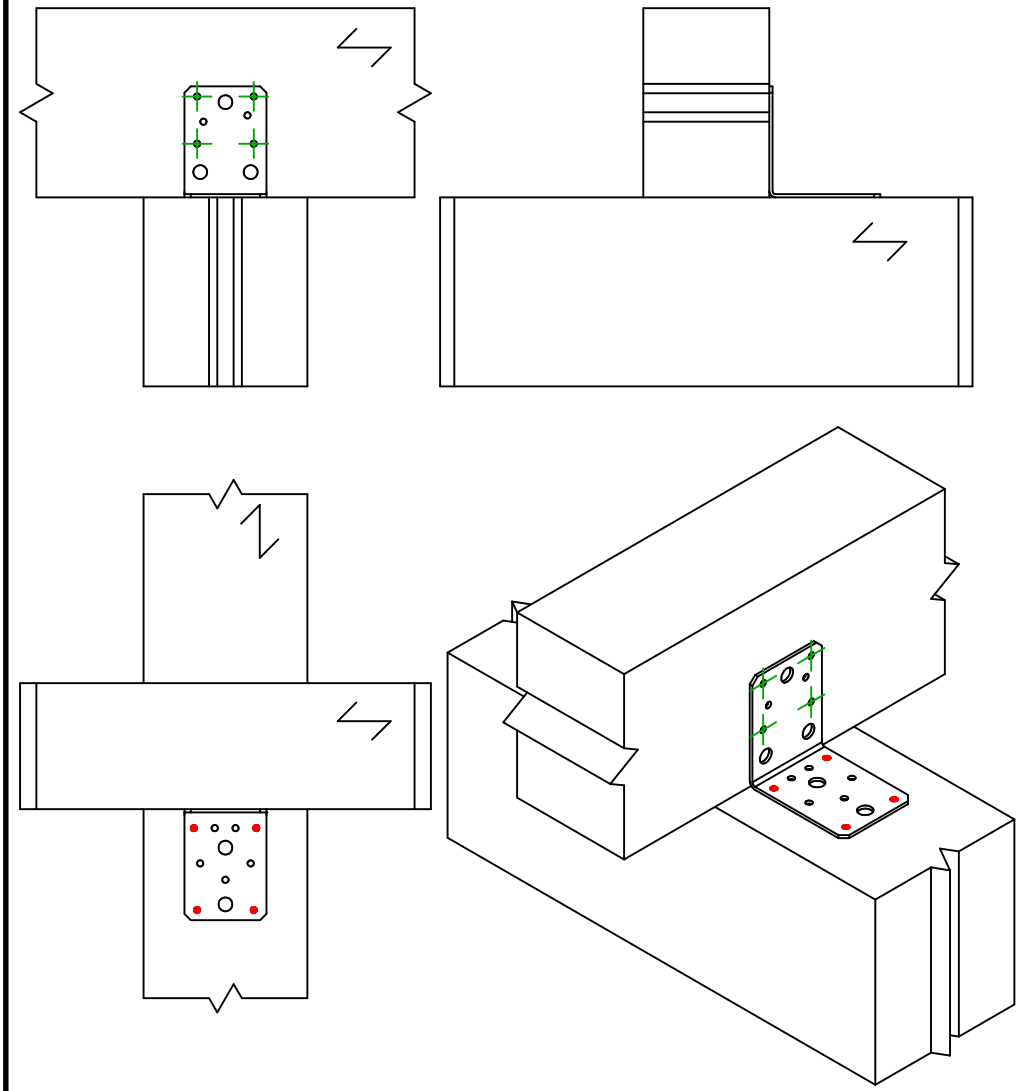
Instalação para 1 esquadro
