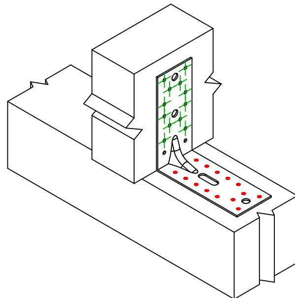
Instalación para 1 escuadra
