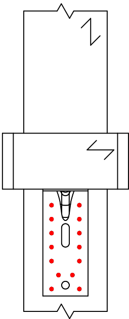
Instalación para 1 escuadra
