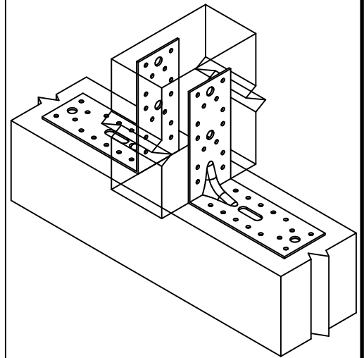
Instalación para 2 escuadras
